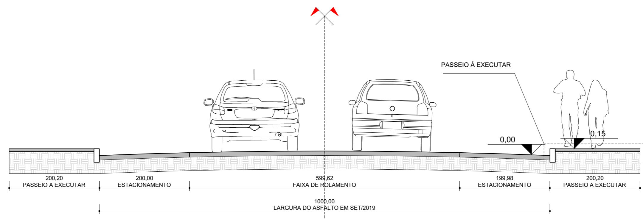
SEÇÃO TRANSVERSAL 1:50
